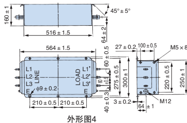
外形图4
