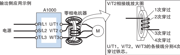
接线图a
