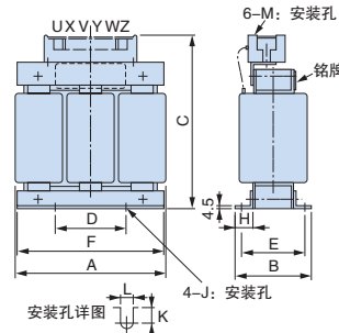
外形图1
