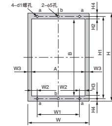
面板加工图1
