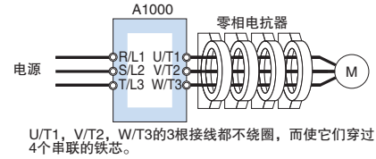
接线图b
