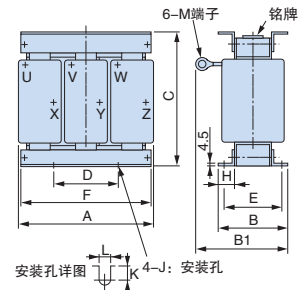
外形图2
