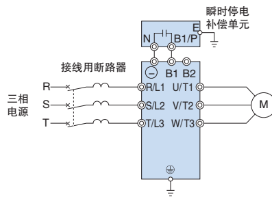
接线图
