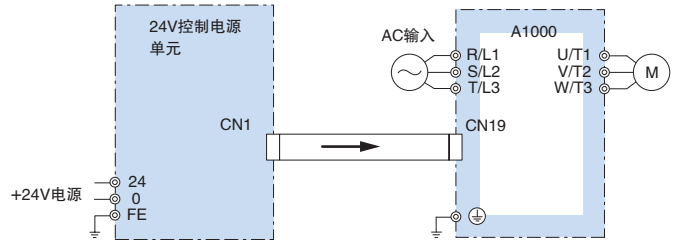
接线图
