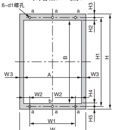
面板加工图4
