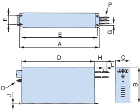
外形图1
