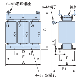
外形图3
