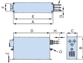
外形图3
