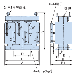
外形图4
